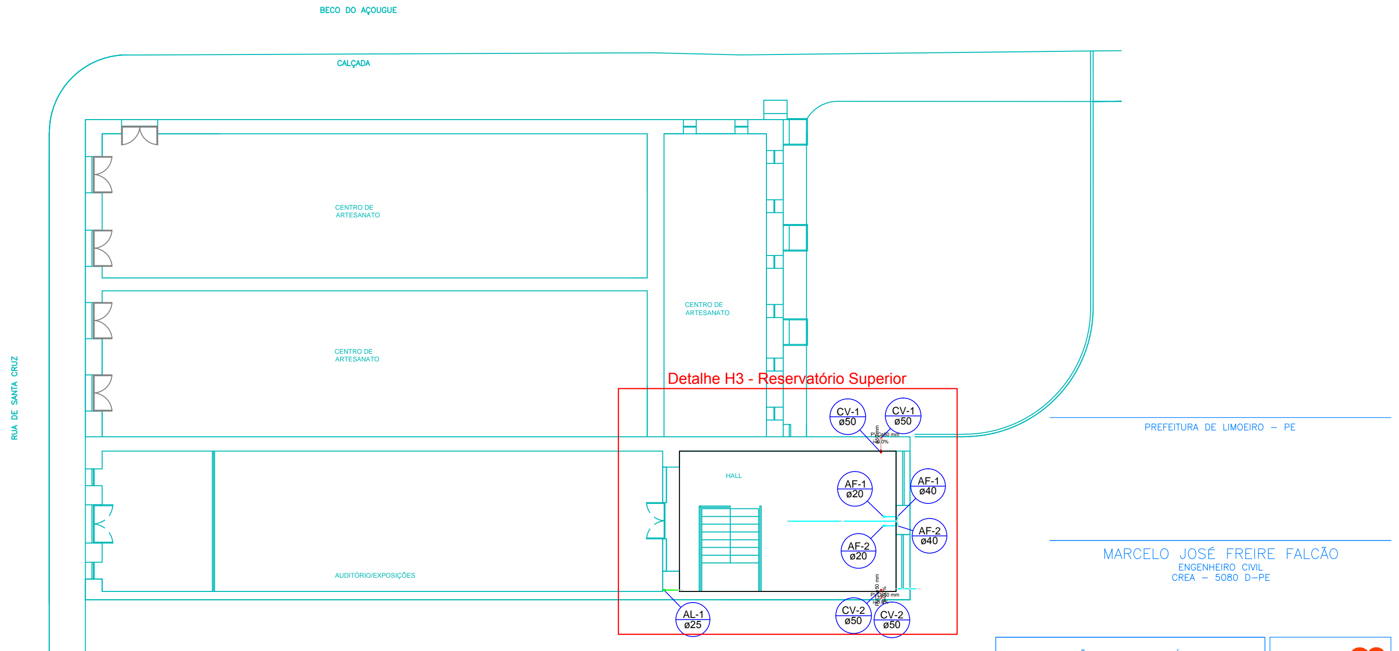
Planta baixa - Pavimento mezanino escala 1:100
