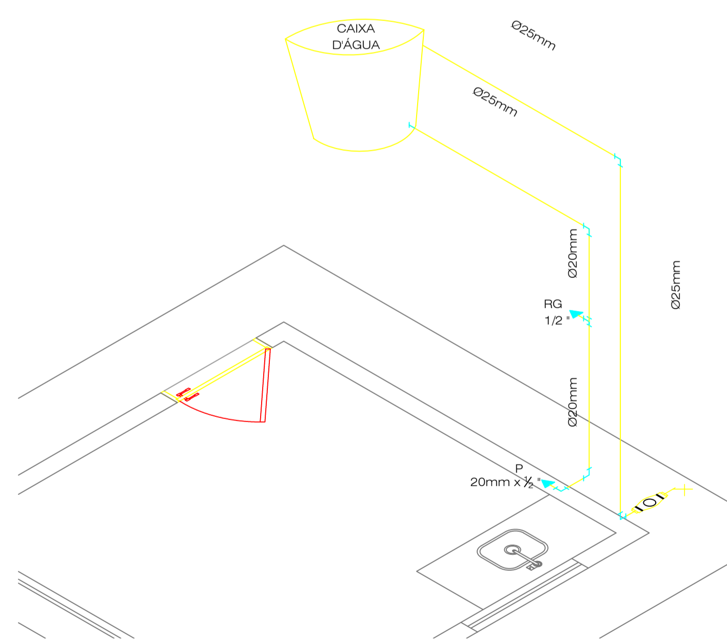
DETALHE ISOMÉTRICO escala 1/25
