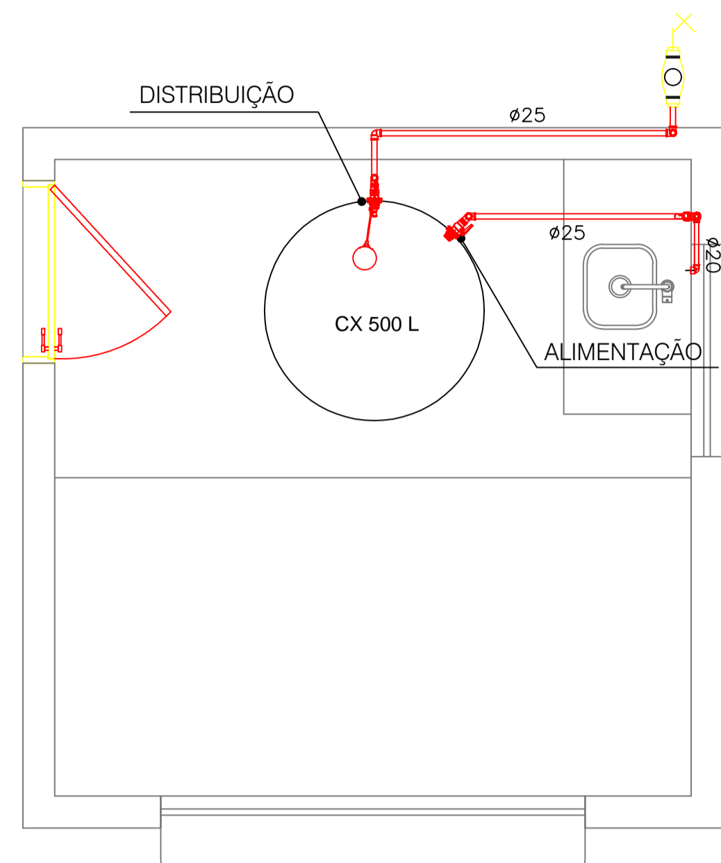
PLANTA BAIXA - ÁGUA FRIA escala 1/25
