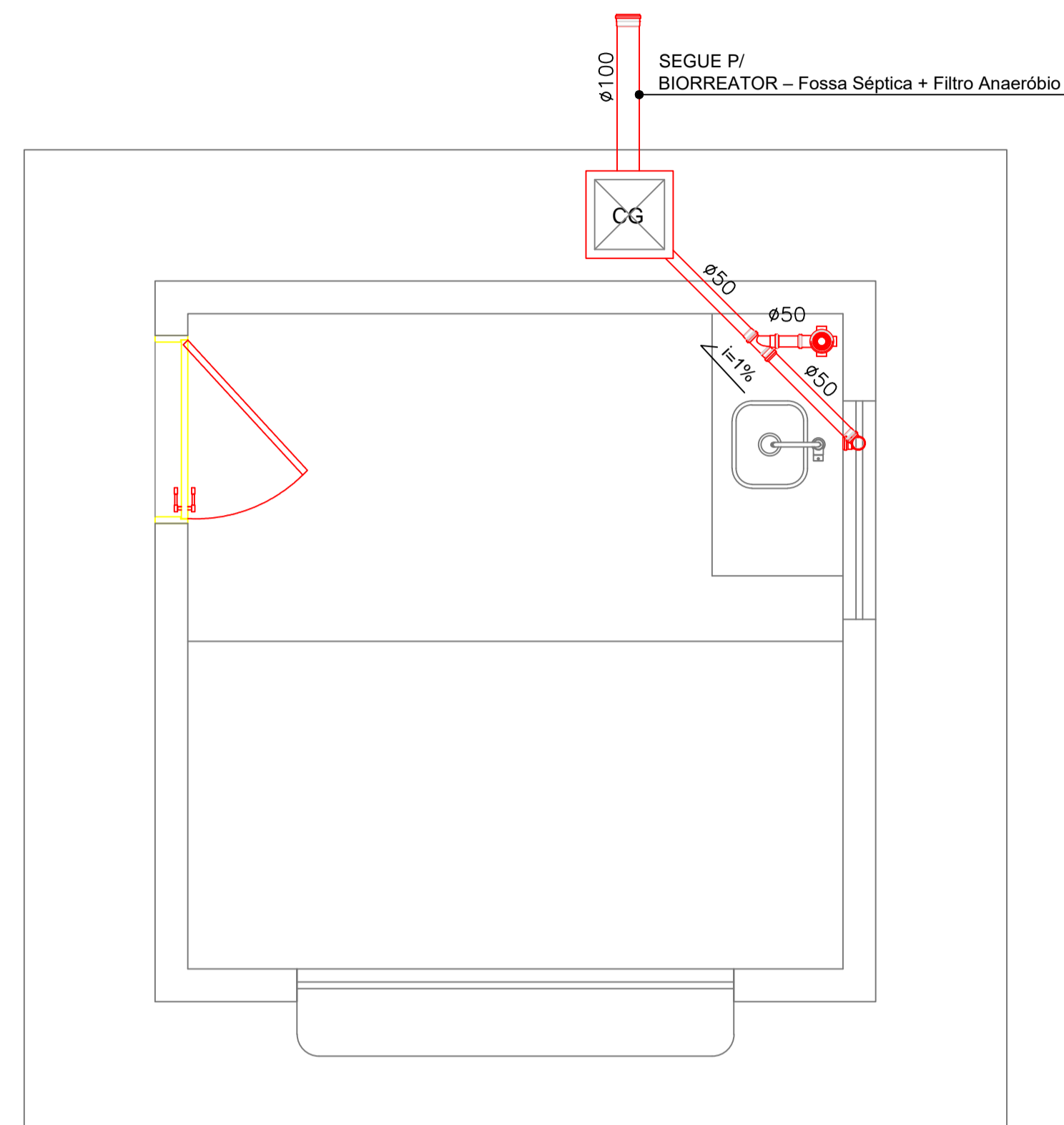
PLANTA BAIXA - ESGOTO escala 1/25
