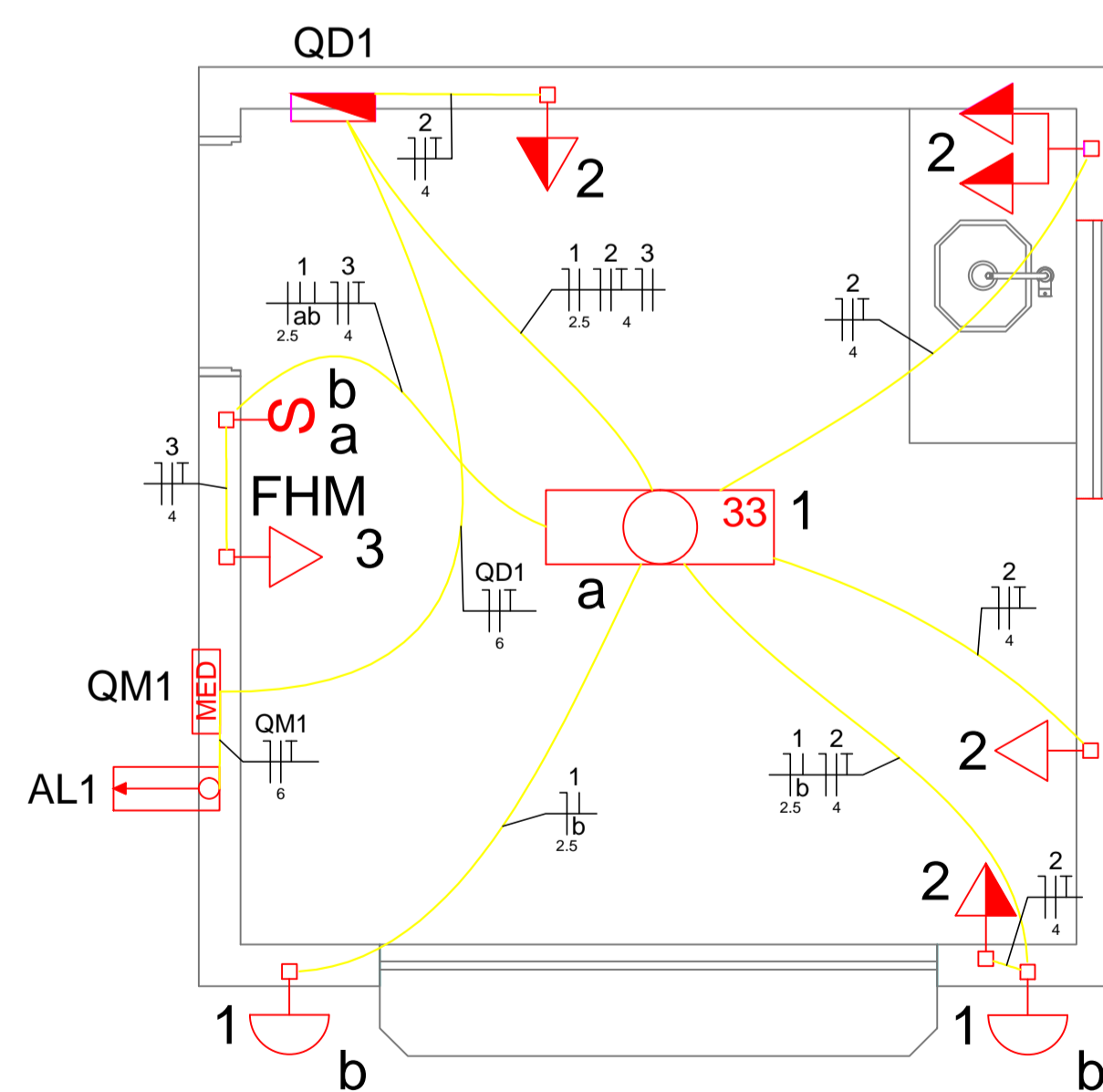
PLANTA BAIXA - ELÉTRICO escala 1/25
