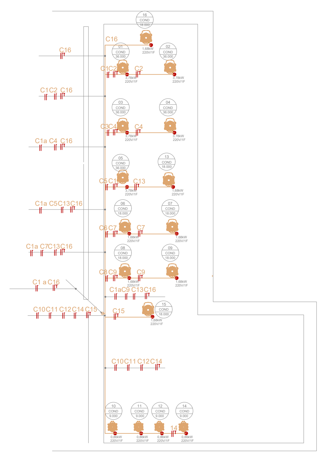
03 Planta baixa laje impermeabilizada - ELÉTRICA Escala 1/100
