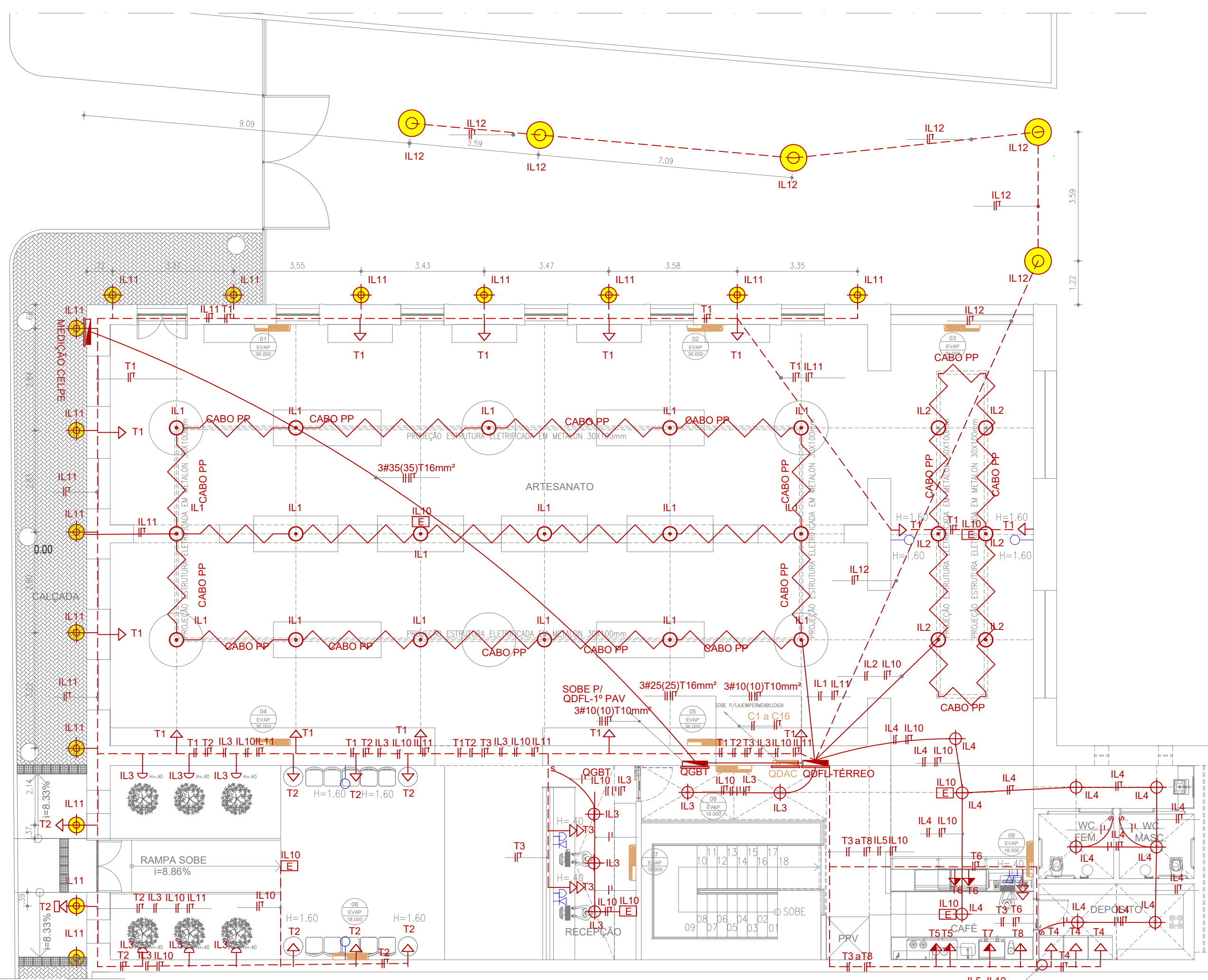
01 Planta baixa pavto térreo - ELÉTRICA Escala 1/700
