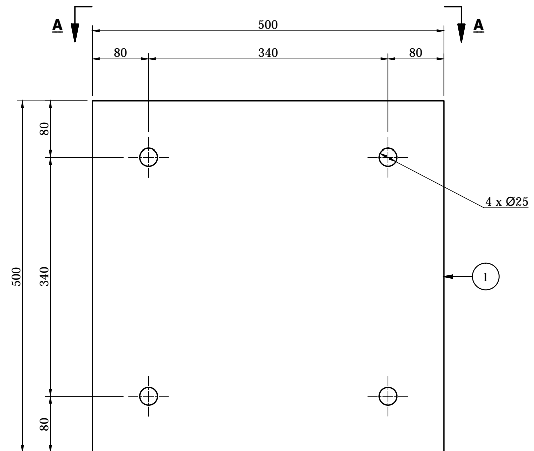
CHAPA DE FUNDAÇÃO ESCALA 1 / 5
