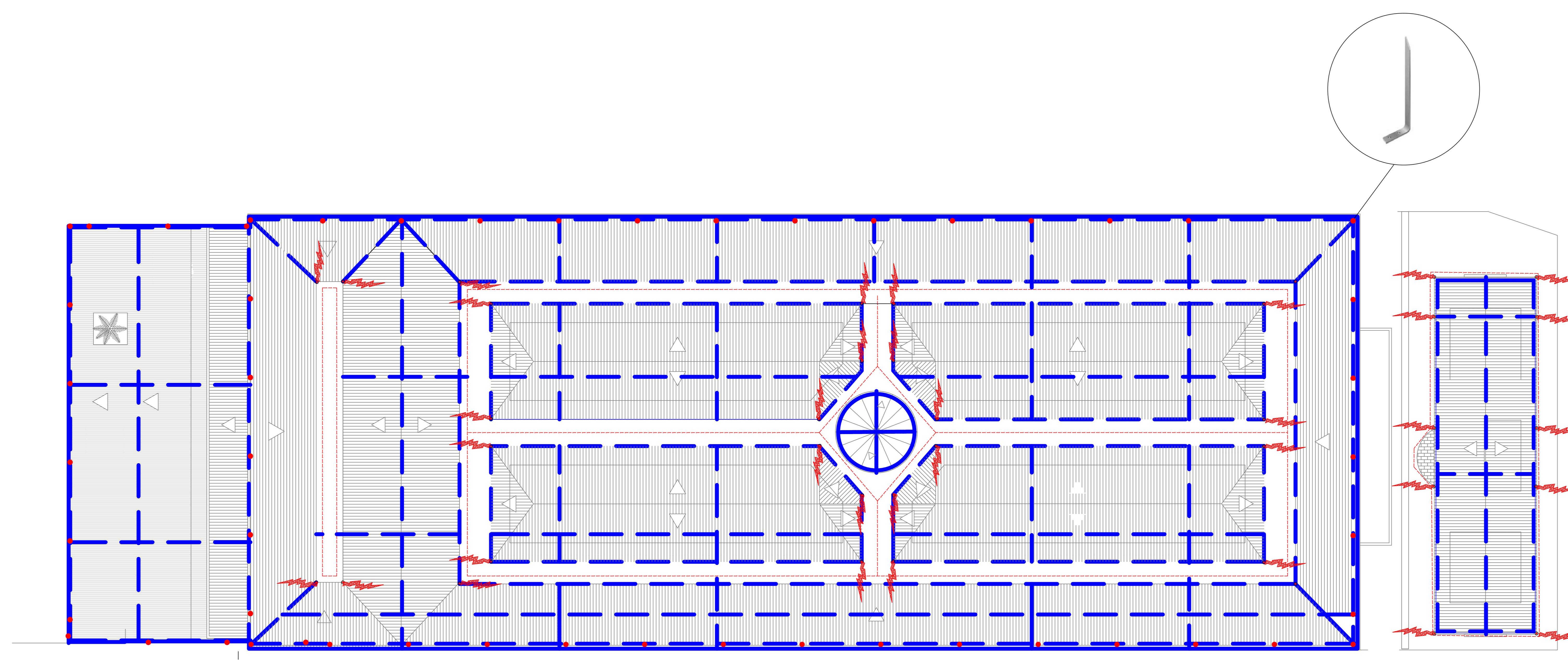
PLANTA DE COBERTA ESCALA: 1/125
